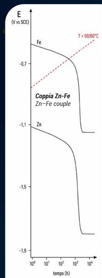
Comportamento della coppia Zn-Fe ad alta temperatura Zn-Fe couple behaviour at high temperature
